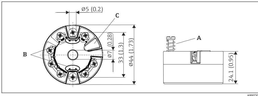
图 6 带螺纹式接线端子的仪表示意图
