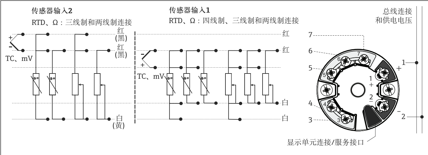
3 模块化变送器的接线端子分配示意图
