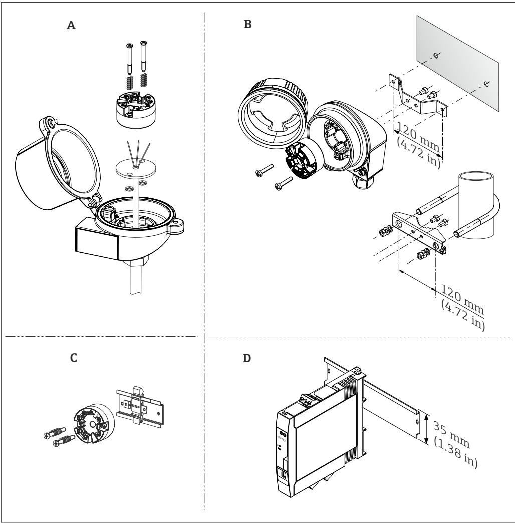
5 变送器的安装方式示意图 A 安装在符合 DIN 50446 标准的表头中(平面)，直接安装在带电缆入口的铠装芯子上(中心孔径: 7 mm (0.28")) B 安装在分体式现场型外壳中，壁式安装或柱式安装 C 使用导轨夹安装在 DIN 导轨上，导轨符合 IEC 60715 标准，TH35 D DIN 导轨型变送器，安装在符合 IEC 60715 标准的 TH35 导轨上
