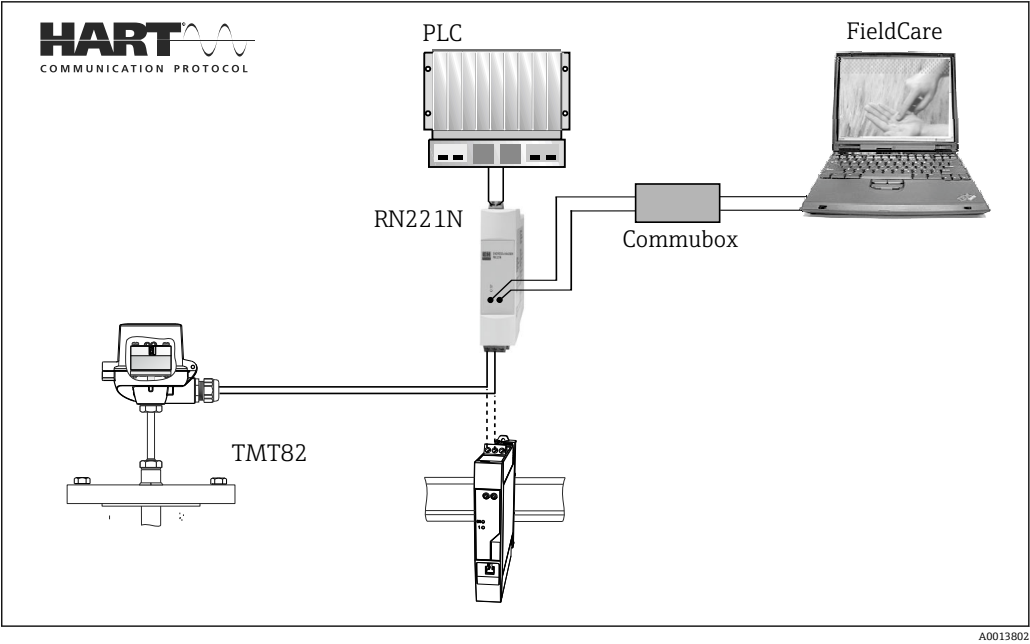
图 2 进行 HART®通信的设备结构示意图
