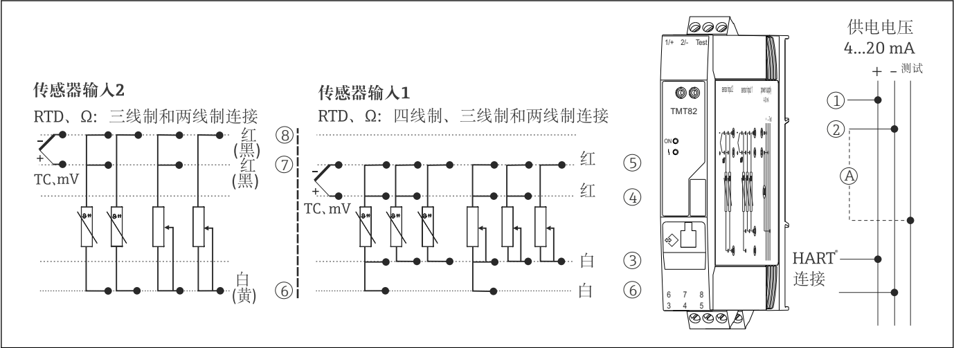
图 4 盘装型变送器的接线端子示意图
