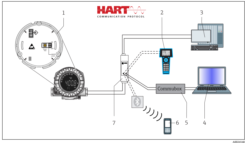
图 9 设备的操作方式
