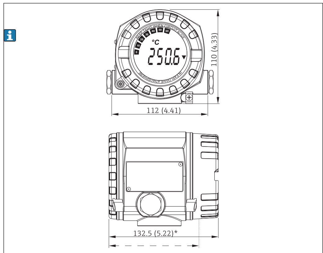
图 7 粉末压铸铝外壳，适用常规应用；或可选不锈钢（316L）外壳
