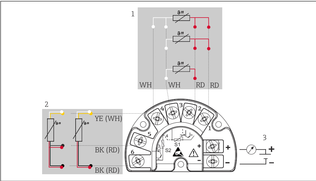
图 2 现场型温度变送器接线：热电阻信号，两路传感器输入 1 传感器输入 1，热电阻信号：两线制、三线制和四线制连接 2 传感器输入 2，热电阻信号：两线制和三线制连接 3 现场型温度变送器电源、4 ... 20 mA 模拟量输出或现场总线连接
