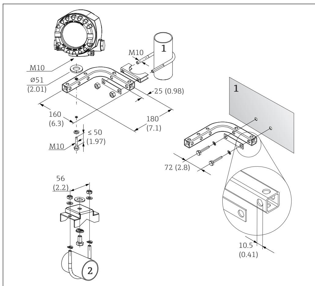
■ 6 使用安装架安装现场型变送器 外形尺寸: mm (in)
