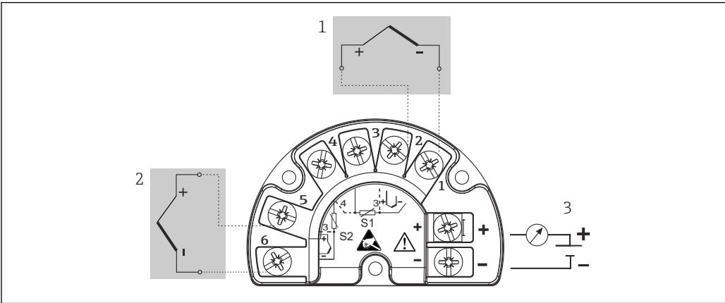
图 3 现场型温度变送器接线：热电偶信号，两路传感器输入 1 传感器输入 1，热电偶信号 2 传感器输入 2，热电偶信号 3 现场型温度变送器电源、4 ... 20 mA 模拟量输出或现场总线连接
