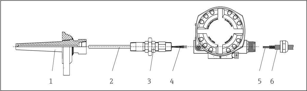
图 5 现场型温度变送器直接安装在传感器上
