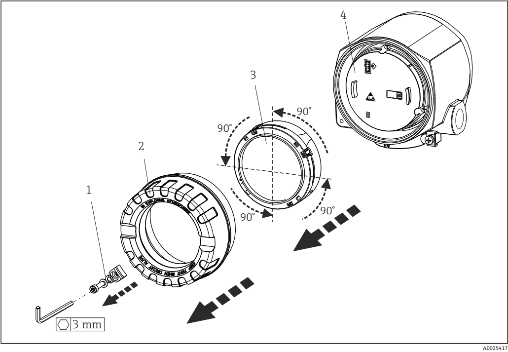
图 7 4 个显示单元固定安装位置，相互间隔 90°
